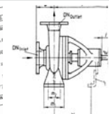
Dimensiones de la bomba conformes a las normas EN733 e ISO2858
