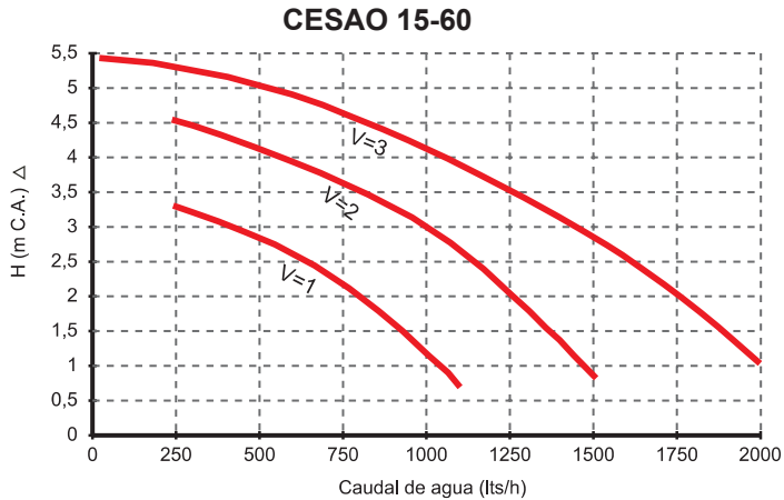
Curva característica del circulador a la salida de la caldera
